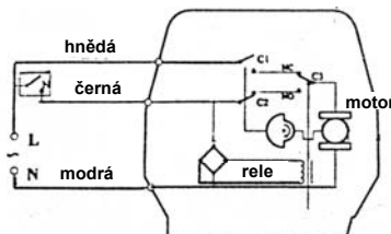
Obrázek 6 – řízení SPST
