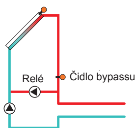
Příklady schémat pro varianty bypassu
