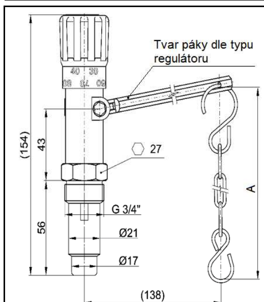
páka RT4
