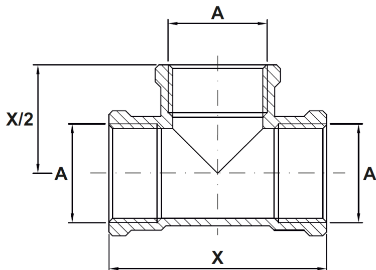
Rozměrové schéma
