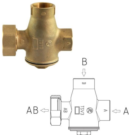
Ventil TSV3B s maticí
